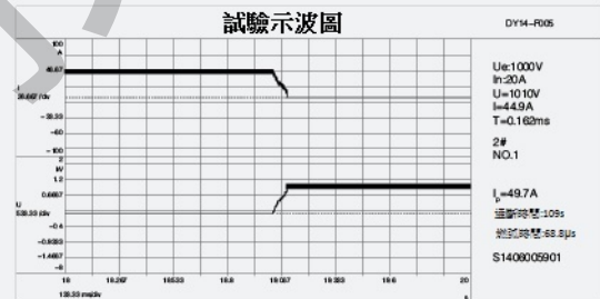
TUV: 1000V DC In20A / 2In:44.9A
