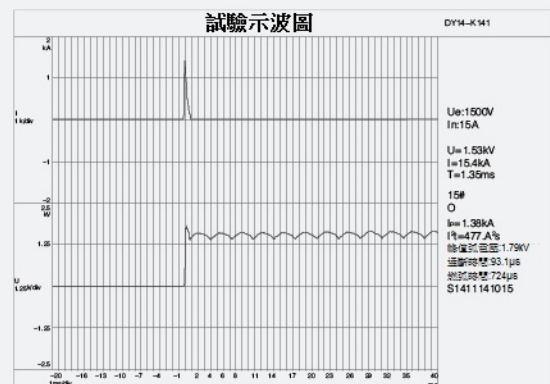
1500V DC In15A / 15.4kA
