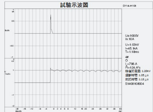
1000V In10A/45.1kA
