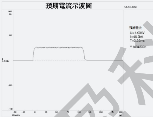
1000V UL In20A/40.3kA 預期電流示波圖
