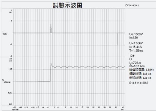
1500V DC In12A / 15.4kA
